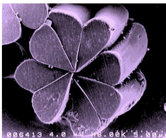
繊維断面図
