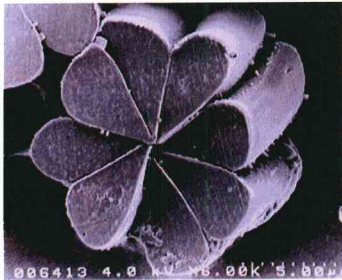
繊維断面図
